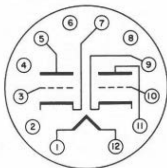
6FJ7 COMPACTRON
