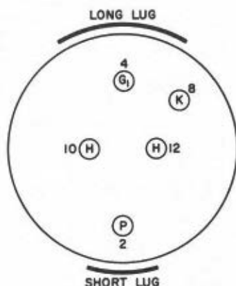
NUVISTOR TRIODE BASE
